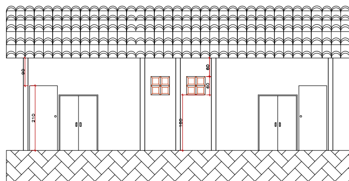
CORTE BB VESTIÁRIOS GARAGEM
