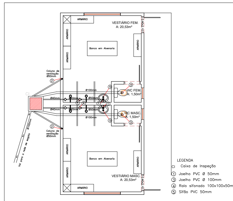
ESGOTO SANITÁRIO VESTIÁRIOS GARAGEM
