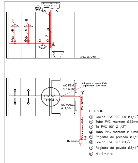
HIDRÁULICO VESTIÁRIOS GARAGEM
