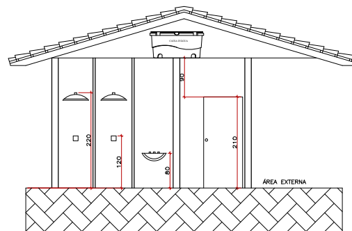
CORTE AA VESTIÁRIOS GARAGEM
