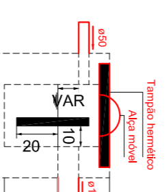
Caixa de gordura Corte 1 - ESC. 1:25
