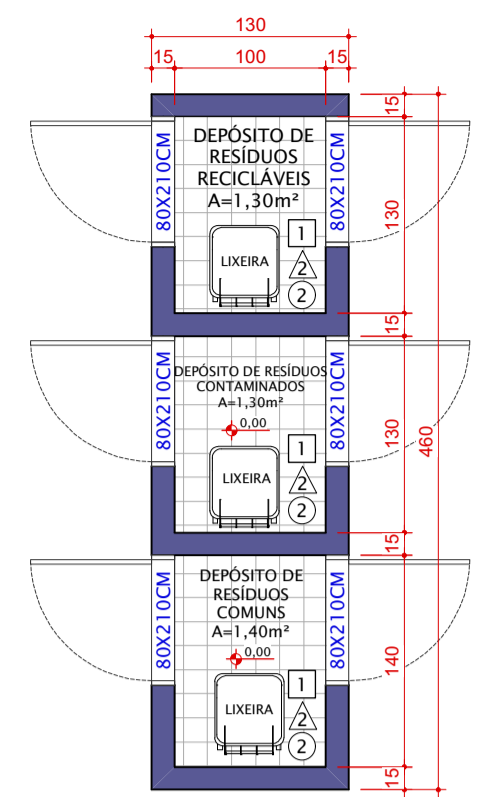
PLANTA BAIXA ABRIGO EXTERNO DE RESÍDUOS SÓLIDOS ESC.: 1/50
