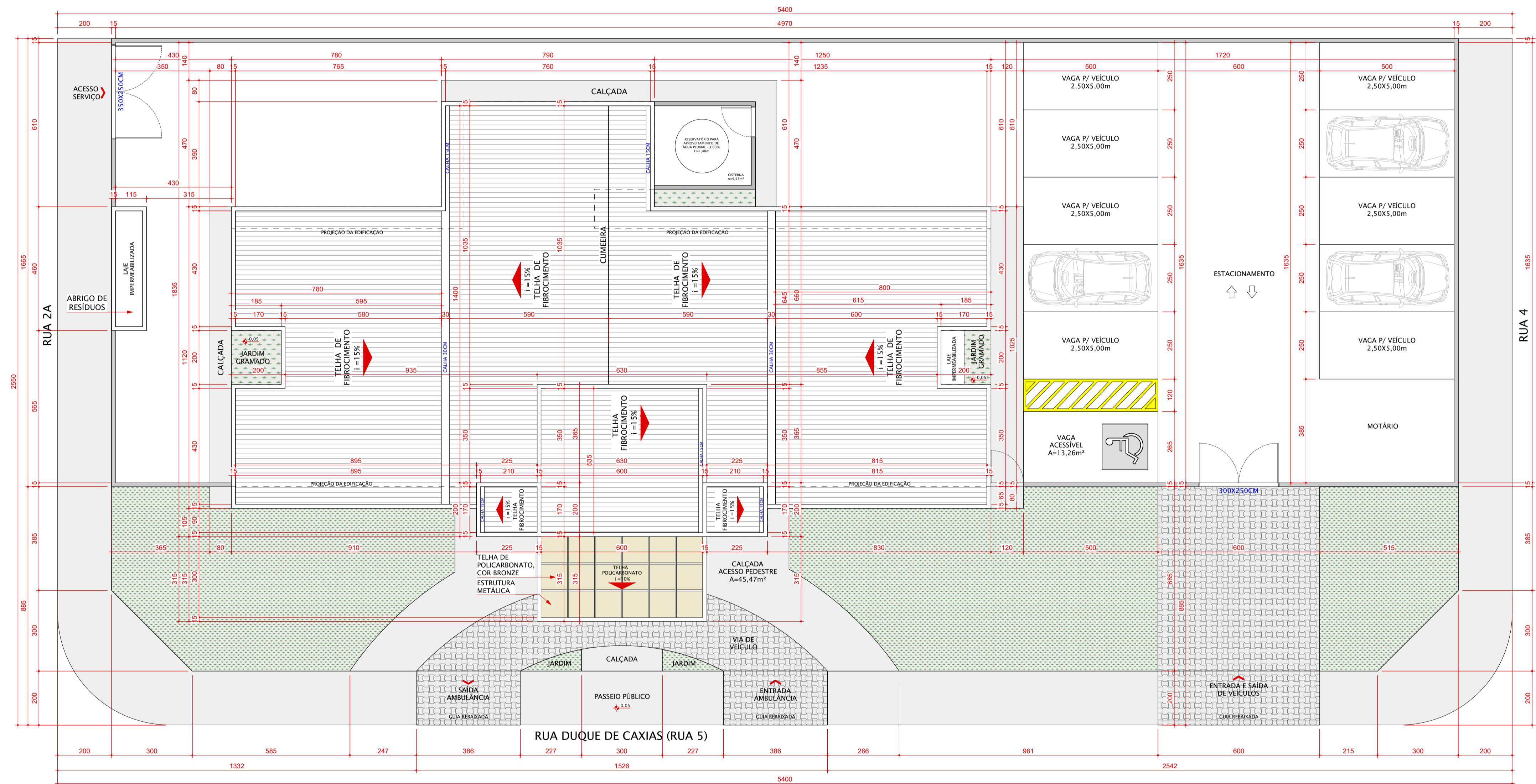
PLANTA DE LOCAÇÃO E COBERTURA ESC.: 1/100
