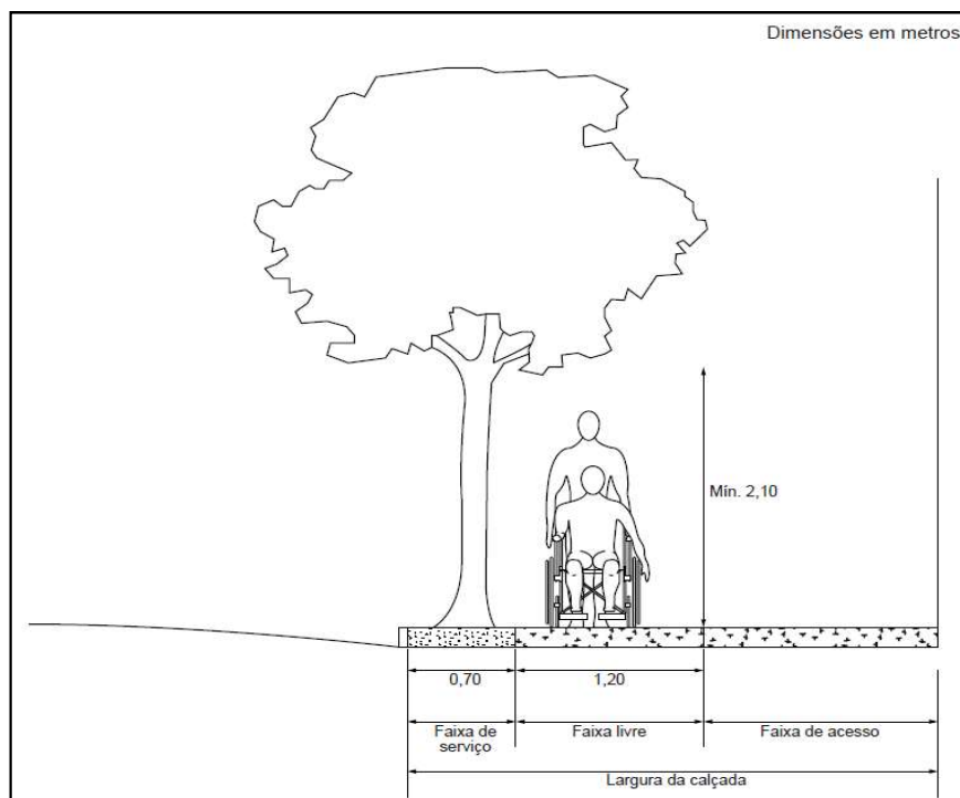
Figura 1 - Faixas de uso da calçada - Corte
