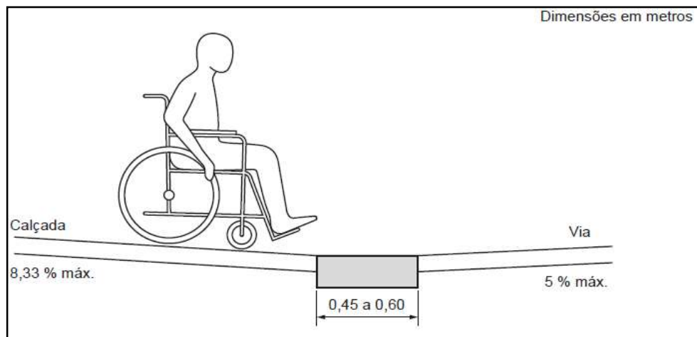
Figura 4 - Faixa de Acomodação para Travessia - Corte
