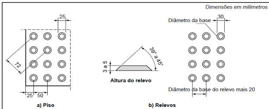
Figura 6 - Sinalização e Relevo Tátil de Alerta Instalados no Piso
