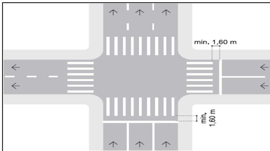
Figura 8 - Dimensões entre LRE e FTP
