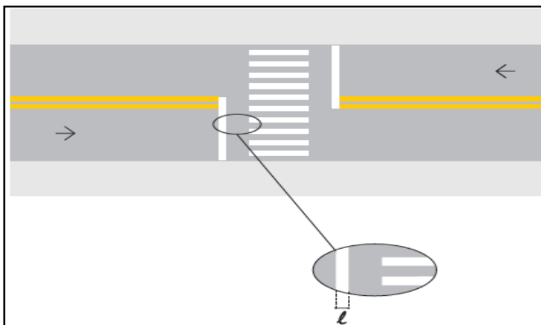
Figura 10 - Dimensões das Linhas da FTP
