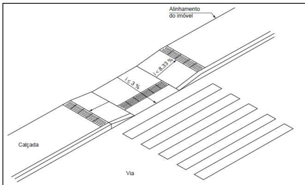
Figura 3 - Rebaixamento de Calçadas
