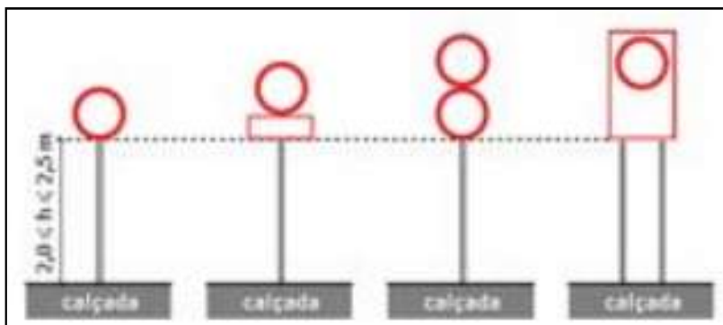
Figura 13 - Limite de altura das placas
