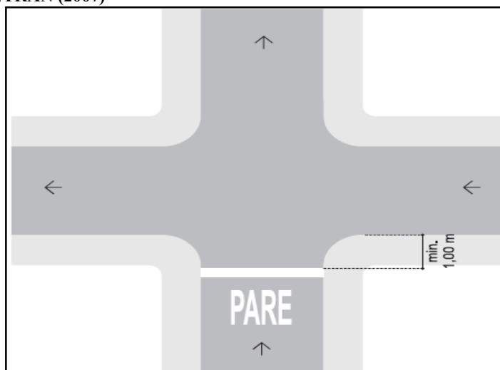
Figura 9 - Dimensões entre LRE e Via
