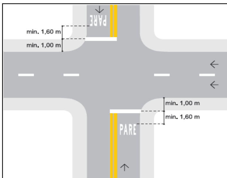
Figura 11 – Dimensões entre o PARE e a LRE
