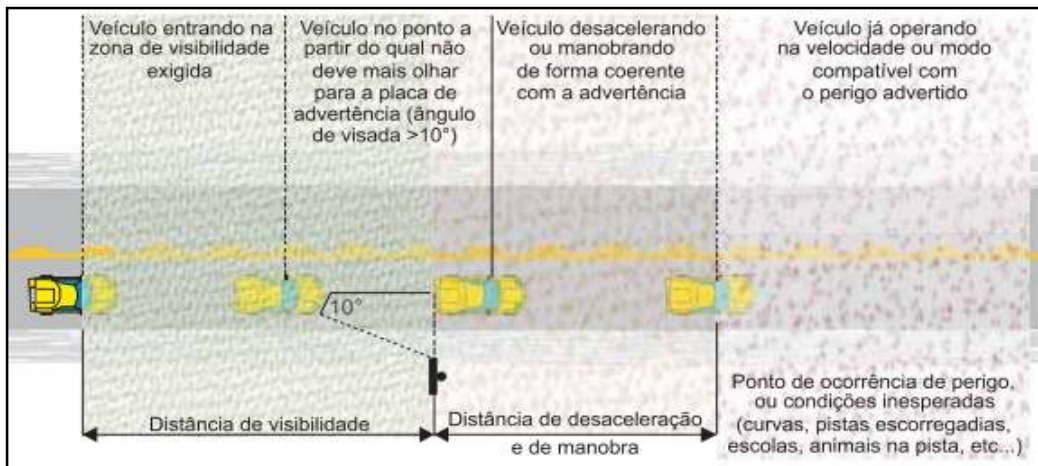
Figura 17 - Posicionamento das Placas de Advertência
