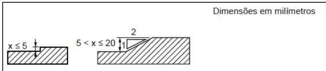
Figura 2 - Tratamento de Desníveis
